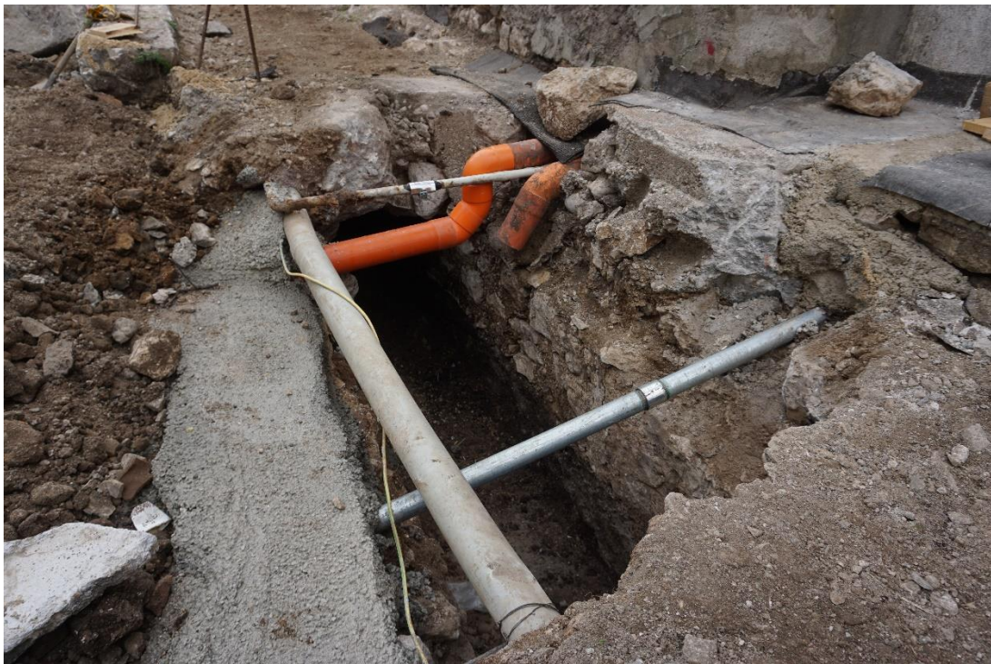
Figura 11. Dettaglio condotta 2.
