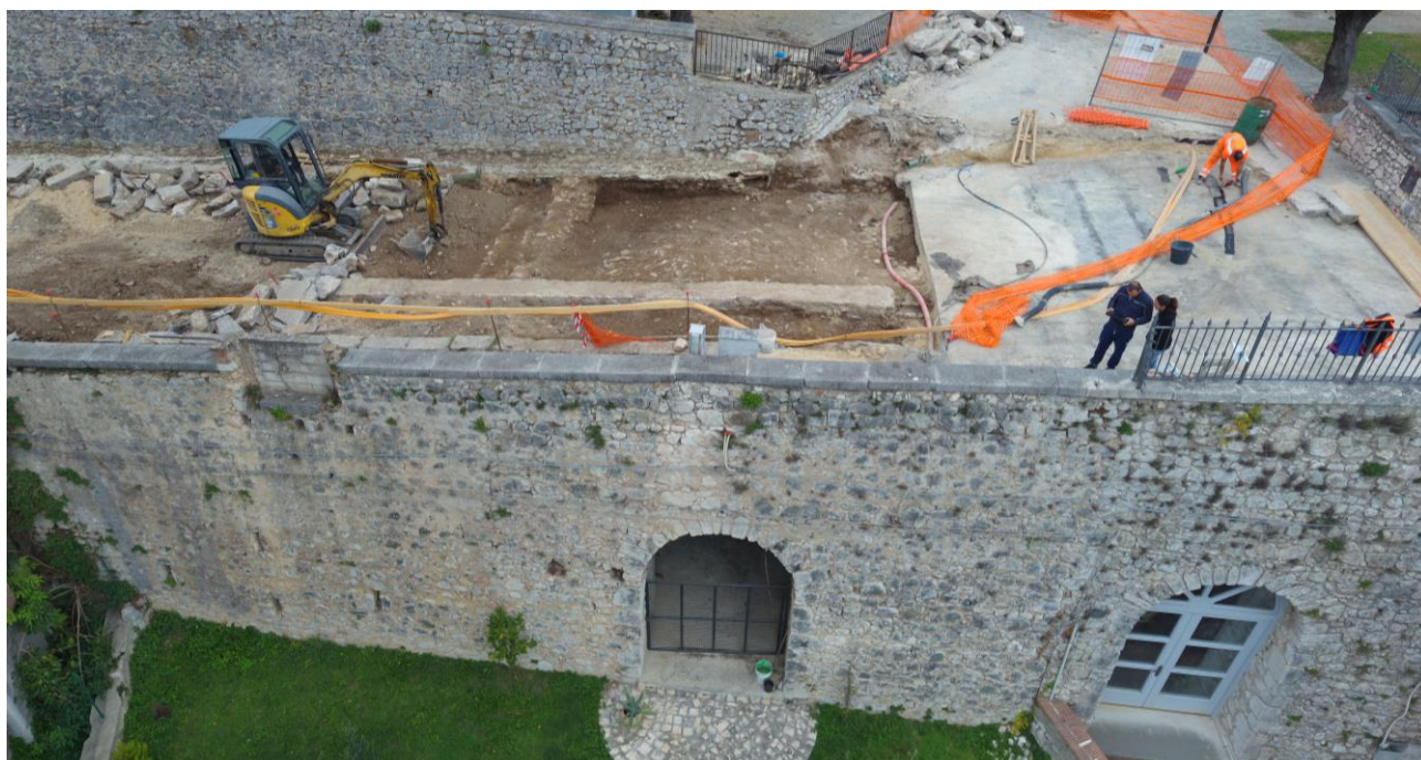
Figura 17. Ambiente voltato a vela via Caserta.
