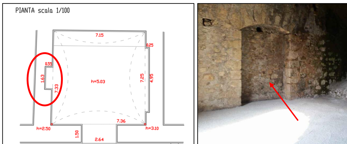
Figura 20. Tamponatura apertura Ovest, ambiente al di sotto di Via Caserta.
